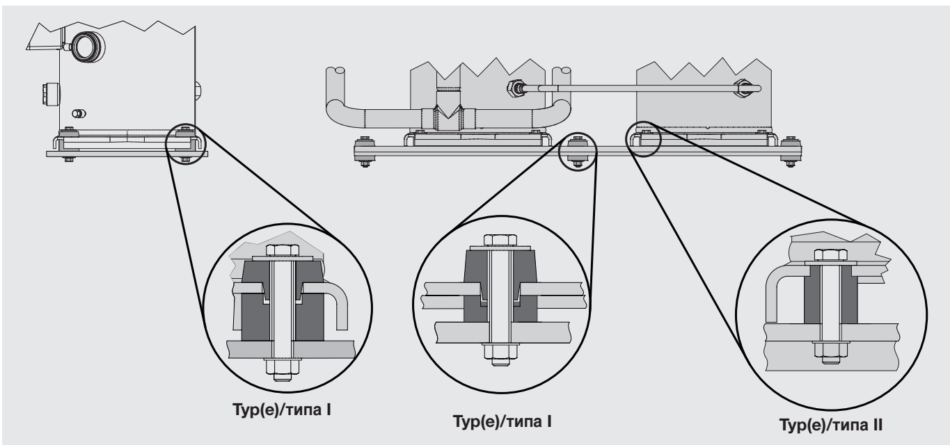
Abb. 2 Schwingungsdämpfer
